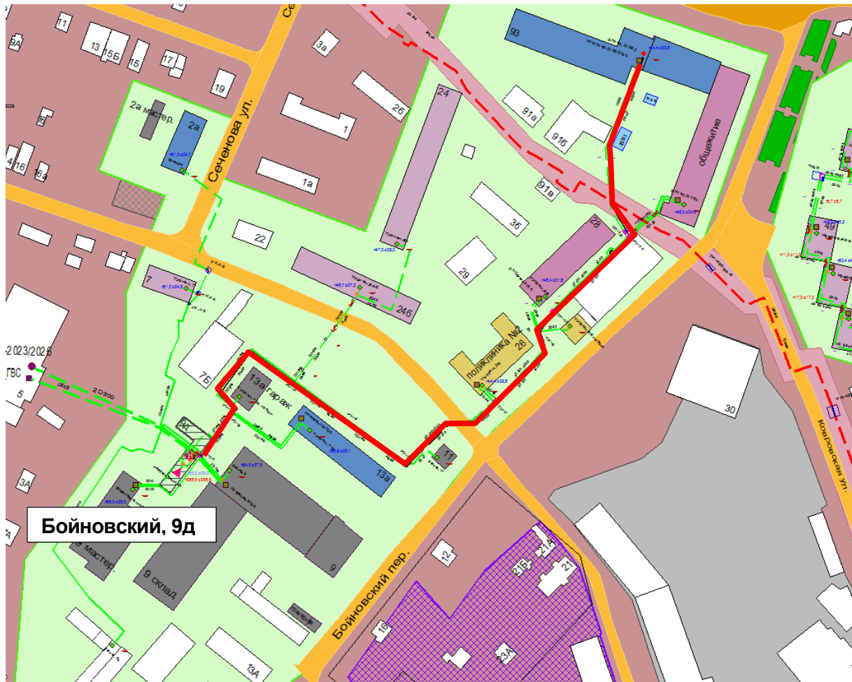
Рисунок Ошибка! Текст указанного стиля в документе отсутствует..13 – Результат гидравлического расчета - расчетный путь теплоносителя от Бойновский, 9д до ПТ-Б.Печер, 93 МВД
