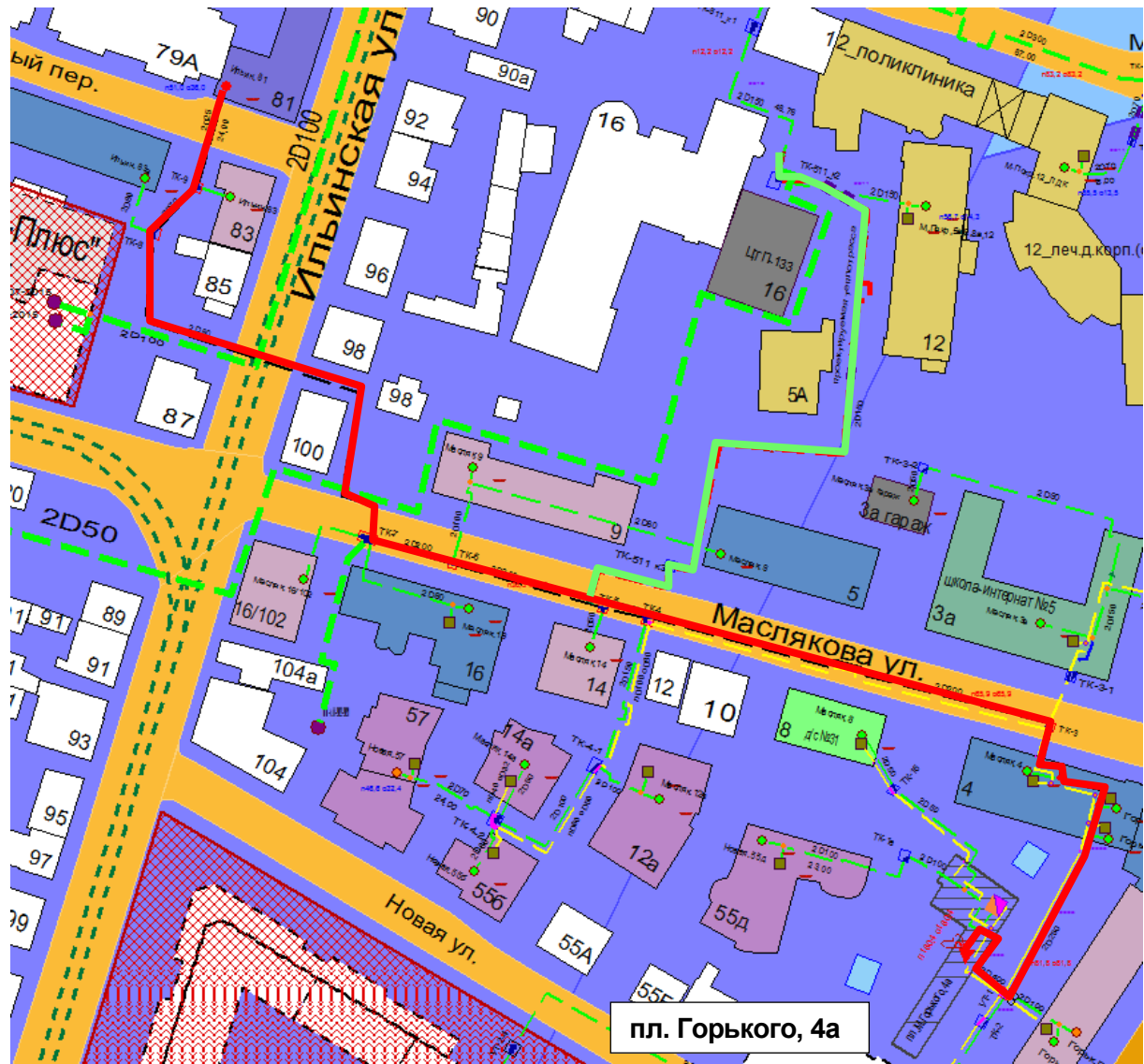
Рисунок Ошибка! Текст указанного стиля в документе отсутствует..45 – Результат гидравлического расчета - расчетный путь теплоносителя от котельной пл. Горького, 4а до ПТ-Ильин,81
