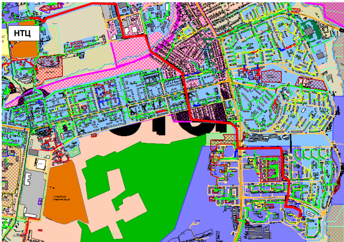
Рисунок Ошибка! Текст указанного стиля в документе отсутствует..33 – Результат гидравлического расчета - расчетный путь теплоносителя от котельной НТЦ до ПТ-Малин,2 пристрой
