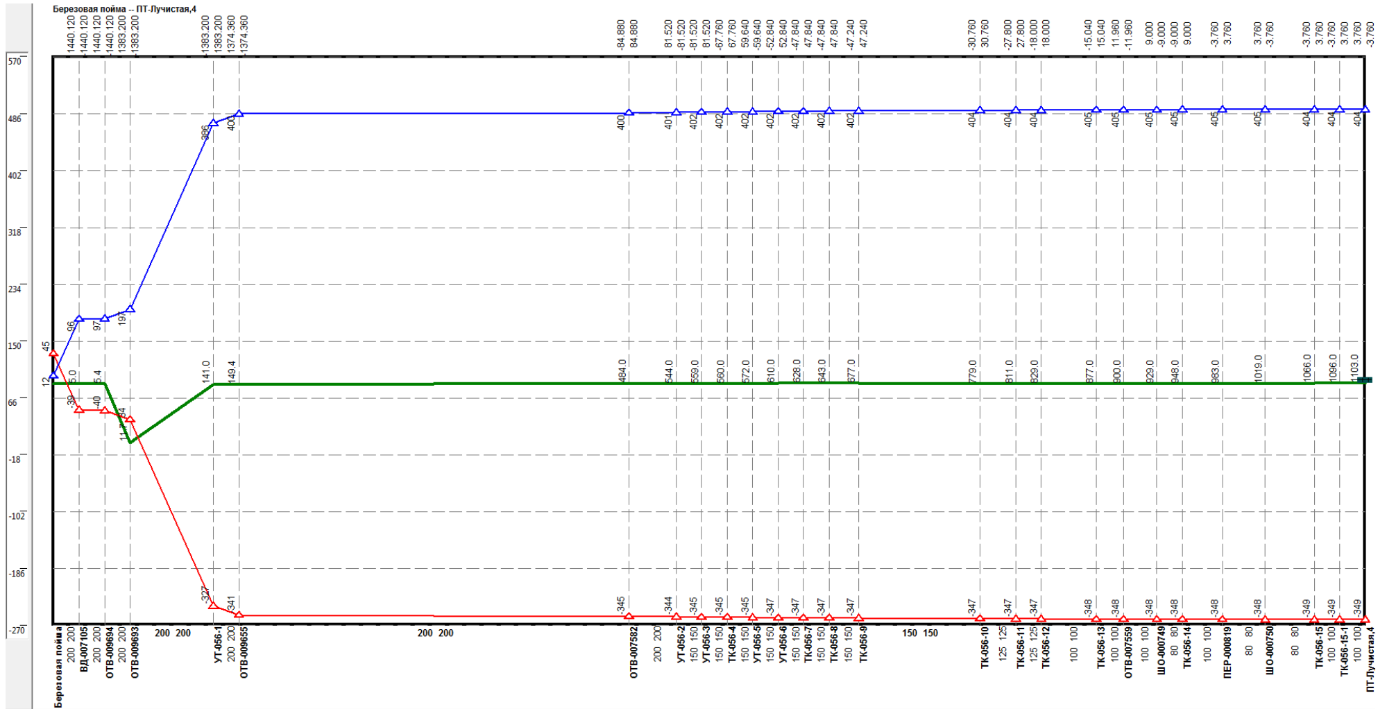
Рисунок Ошибка! Текст указанного стиля в документе отсутствует..16 –Результат гидравлического расчета - график гидравлических режимов по пути теплоносителя от котельной Березовая пойма до ПТ-Лучистая, 4
