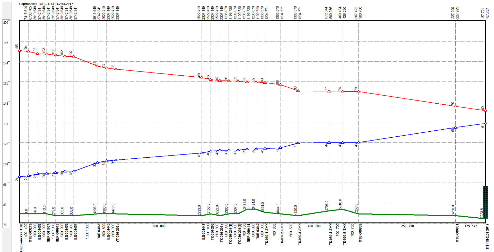
Рисунок Ошибка! Текст указанного стиля в документе отсутствует..4 –Результат гидравлического расчета - график гидравлических режимов по пути теплоносителя от СЭЦ до ПТ-ПП-2.64-2017
