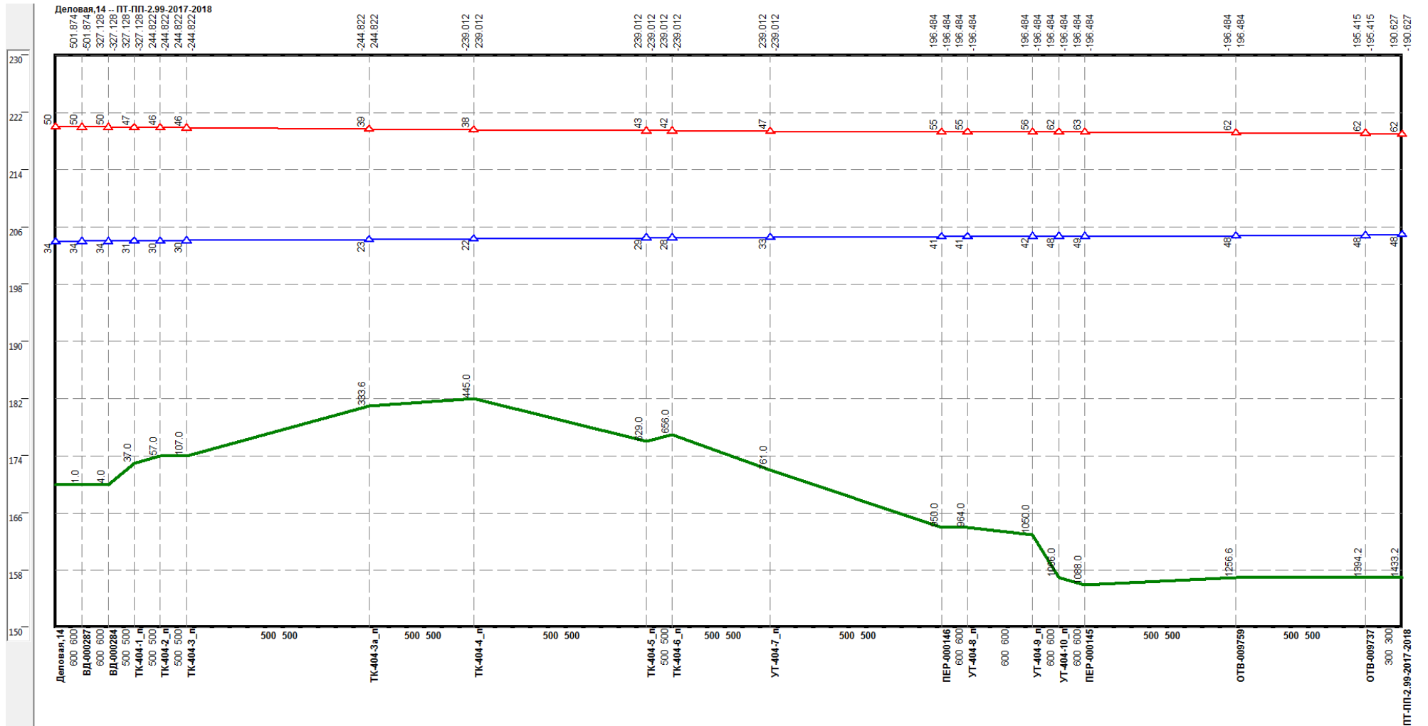
Рисунок Ошибка! Текст указанного стиля в документе отсутствует..20 –Результат гидравлического расчета - график гидравлических режимов по пути теплоносителя от котельной Деловая, 14 до ПТ-ПП-2.99-2017-2018.
