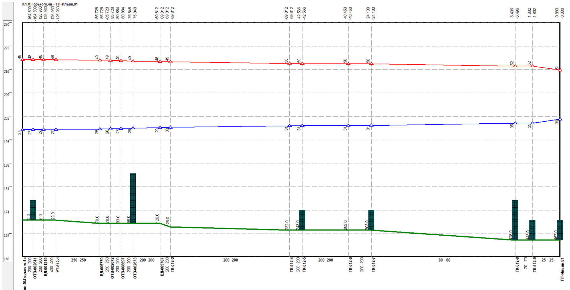
Рисунок Ошибка! Текст указанного стиля в документе отсутствует..46 –Результат гидравлического расчета - график гидравлических режимов по пути теплоносителя от котельной пл. Горького, 4а до ПТ-Ильин,81
