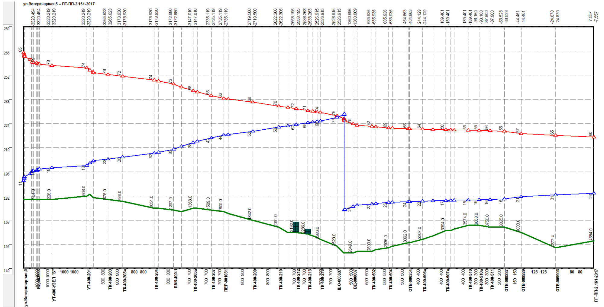
Рисунок Ошибка! Текст указанного стиля в документе отсутствует..38 –Результат гидравлического расчета - график гидравлических режимов по пути теплоносителя от котельной НТЦ до ОТВ-009903
