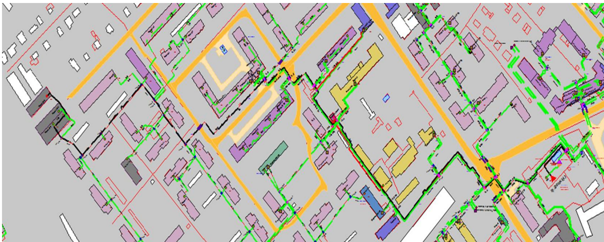
Рисунок Ошибка! Текст указанного стиля в документе отсутствует..49 - Результат гидравлического расчета - расчетный путь теплоносителя от котельной пр . Союзный, 43 до ПТ-Комин,256 э2
