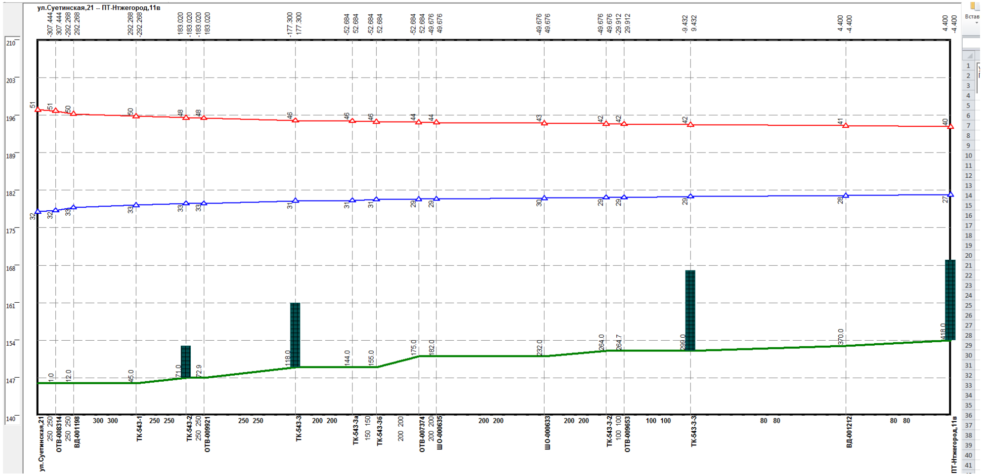
Рисунок Ошибка! Текст указанного стиля в документе отсутствует..10 –Результат гидравлического расчета - график гидравлических режимов по пути теплоносителя от котельной Суетенская, 21 до ПТ-Нтжегород, 11в
