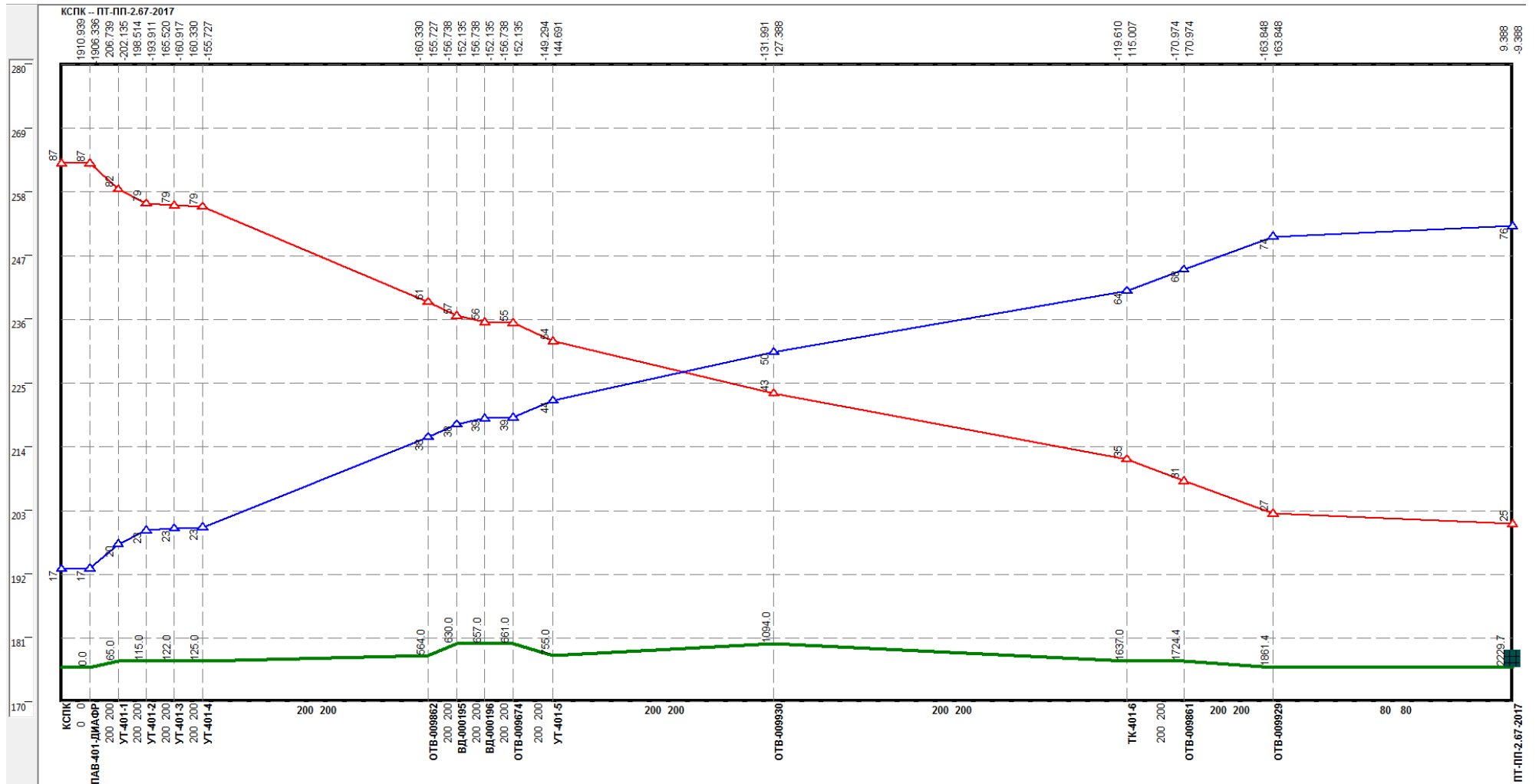
Рисунок Ошибка! Текст указанного стиля в документе отсутствует..52 –Результат гидравлического расчета - график гидравлических режимов по пути теплоносителя от котельной ул. Родионова, 194б до ПТ-ПП-2.67-2017
