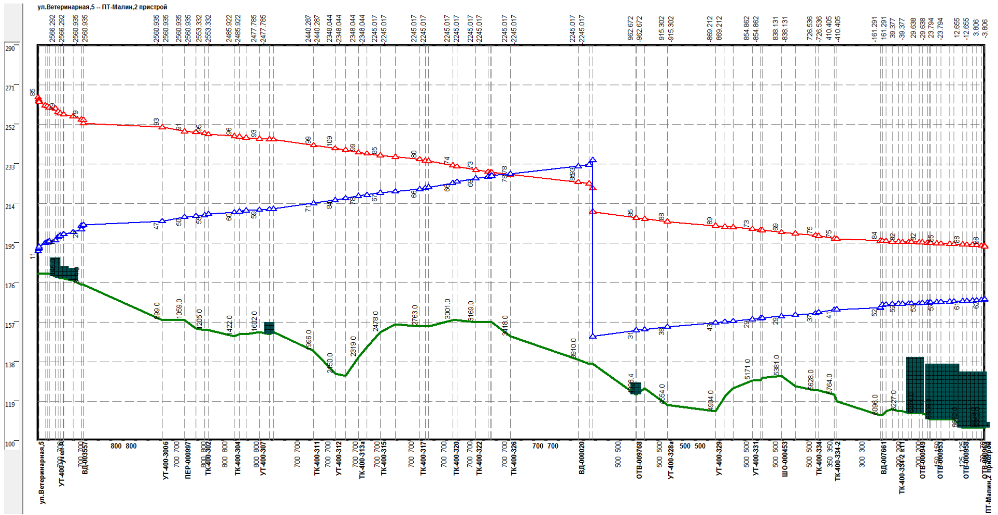
Рисунок Ошибка! Текст указанного стиля в документе отсутствует...34 –Результат гидравлического расчета - график гидравлических режимов по пути теплоносителя от котельной НТЦ до ПТ-Малин,2 пристрой
