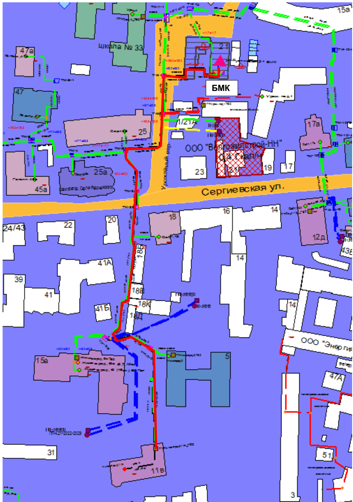
Рисунок Ошибка! Текст указанного стиля в документе отсутствует..9 – Результат гидравлического расчета - расчетный путь теплоносителя от котельной Суетенская, 21 до ПТ-Нтжегород,11в
