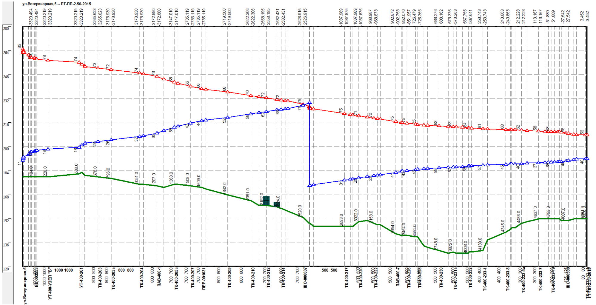
Рисунок Ошибка! Текст указанного стиля в документе отсутствует..36 –Результат гидравлического расчета - график гидравлических режимов по пути теплоносителя от котельной НТЦ до ПТ-В.Волж.наб, проект
